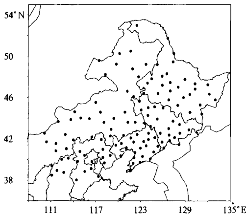
图 1 研究区域 123 个站点分布
