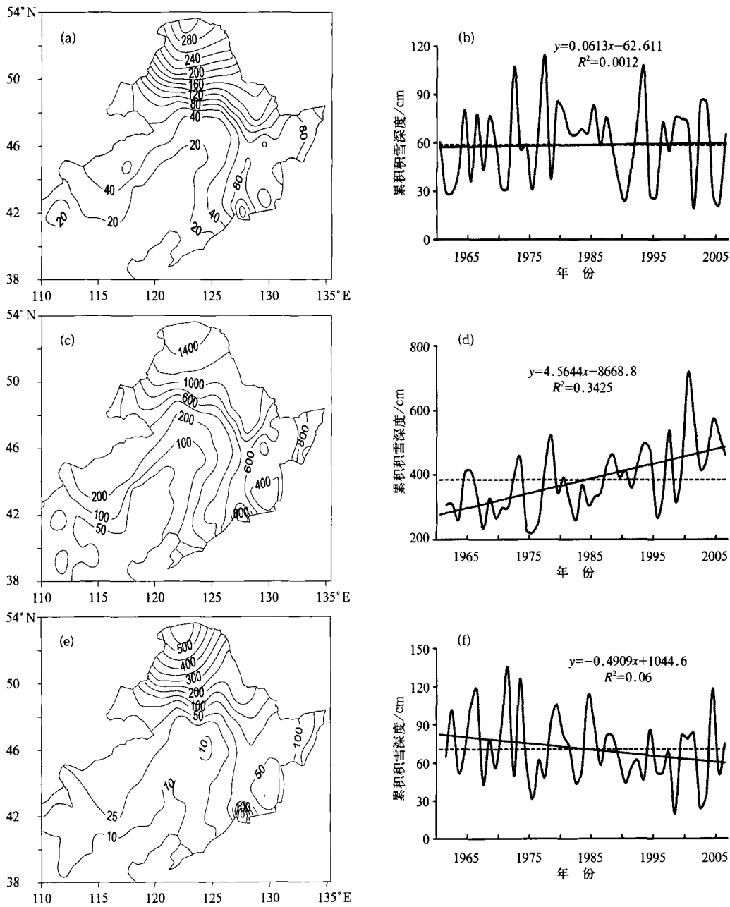
图 5 东北地区秋季(a,b),冬季(c,d)和春季(e,f)累积积雪深度分布 (单位:cm)及其年际变化(说明同图 4)
