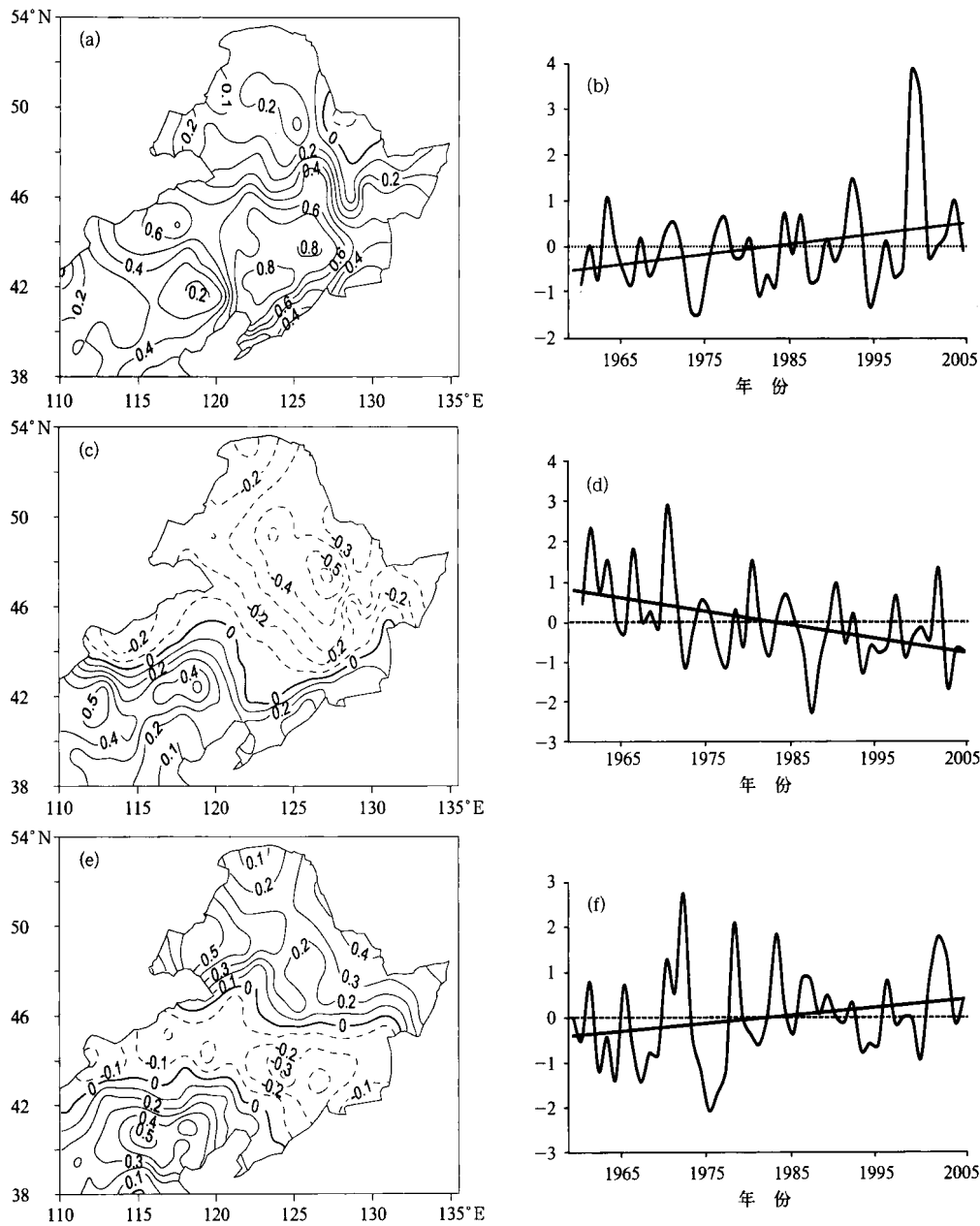
图 7 累积积雪深度的第一(a,b),第二(c,d)和第三(e,f)载荷向量及其所对应的时间系数 Fig. 7 The first (a,b), second (c,d) and third (e,f) loading eigenvectors and the corresponding temporal coefficients of cumulative snow depth
